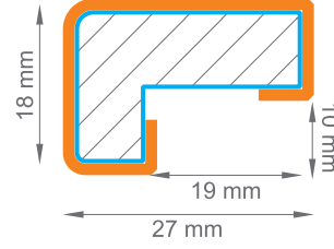
42 mm Kanat İçin Cam Çıtası / Glass Profile for 42 mm Wing
