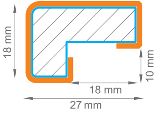
40 mm Kanat İçin Cam Çıtası / Glass Profile for 40 mm Wing
