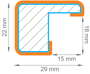
40 mm Kanat İçin Cam Çıtası / Glass Profile for 40 mm Wing
