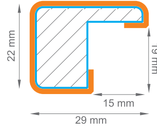
42 mm Kanat İçin Cam Çıtası / Glass Profile for 42 mm Wing
